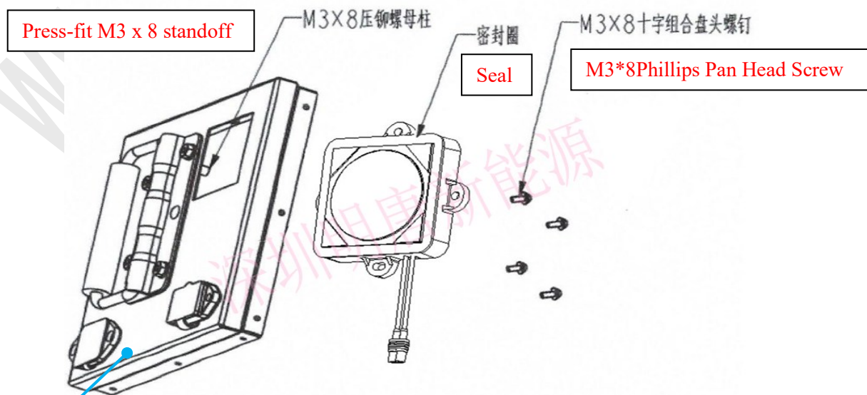
安装参考图 Installation Reference Diagram
