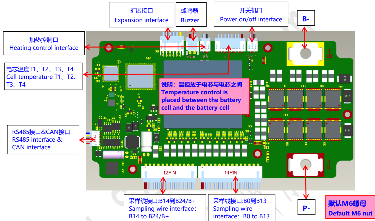
BM569KO-V02接插件详细型号说明
